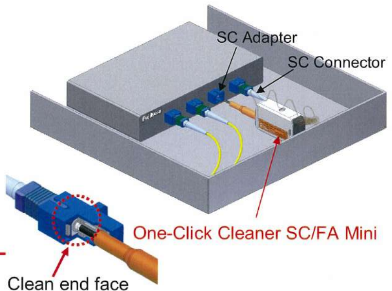
One-Click Cleaner SC/FA Mini
